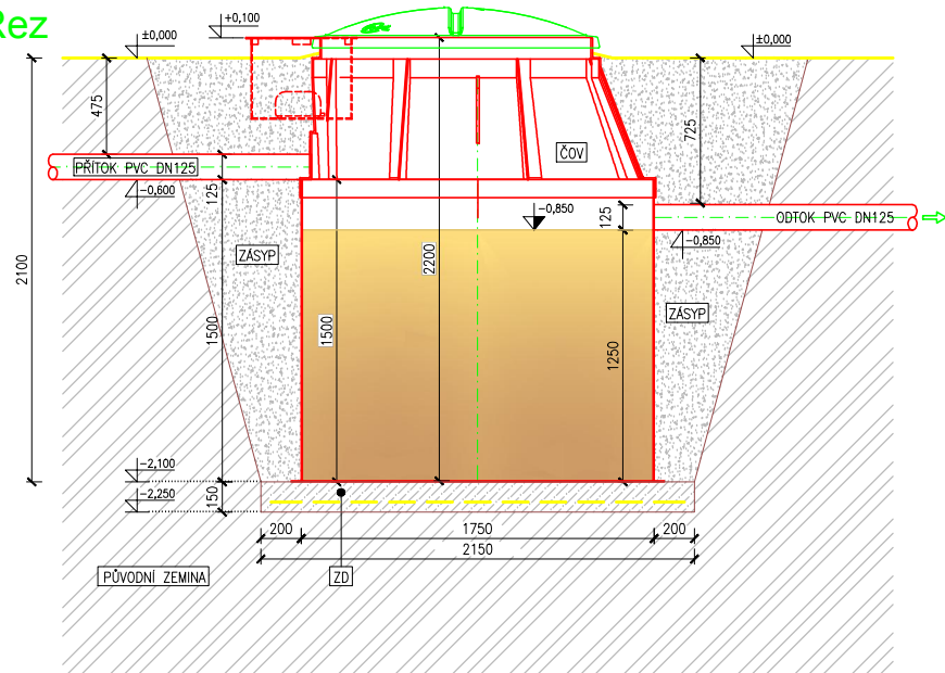
Řez
